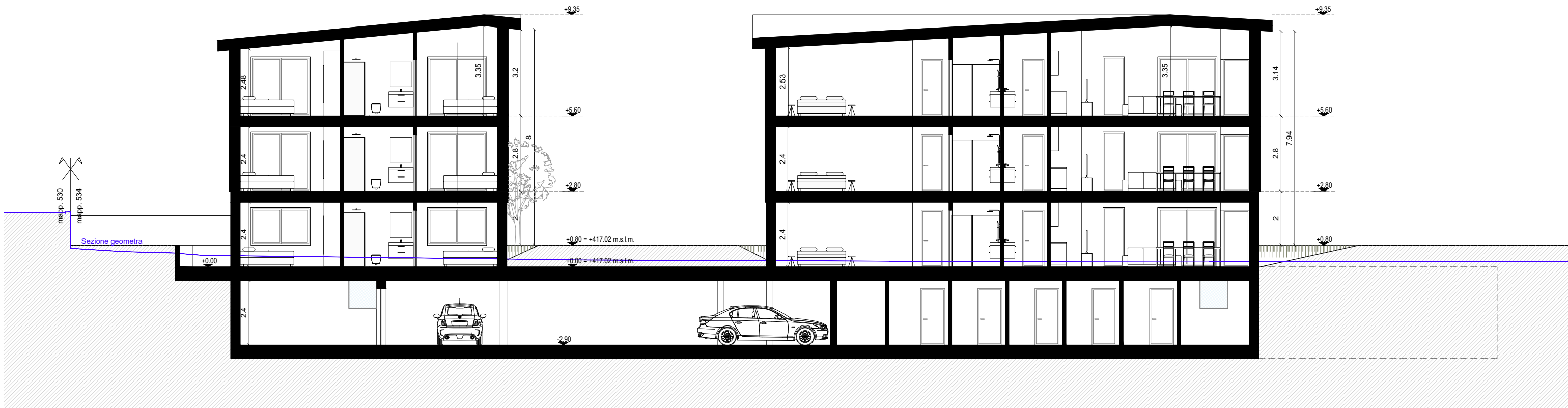
Sezione A-A
