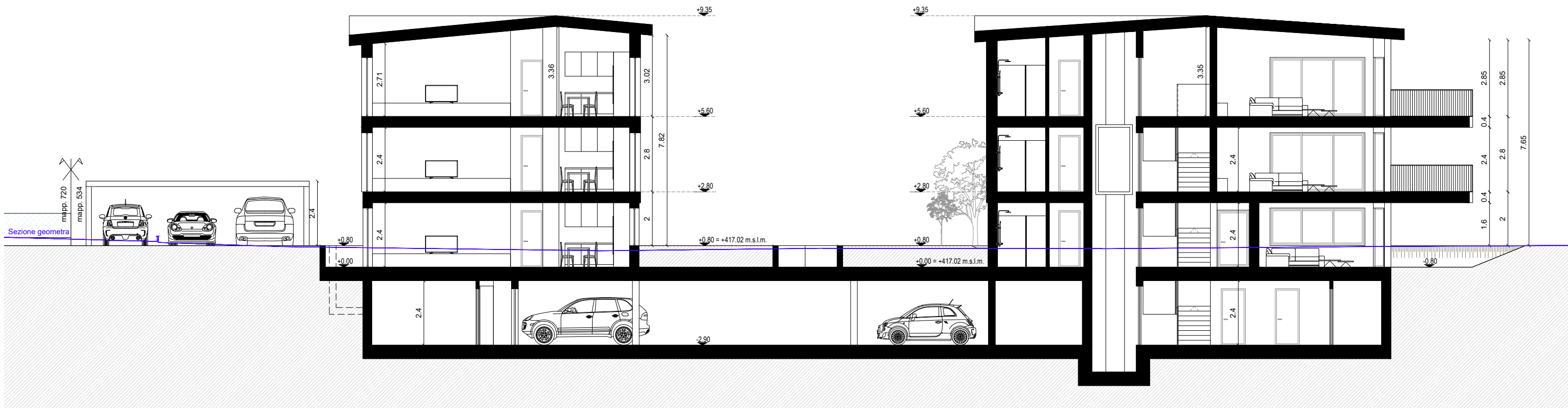
Sezione B-B
